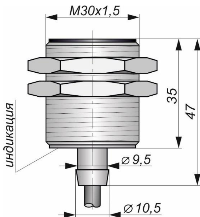
Габаритный чертеж
